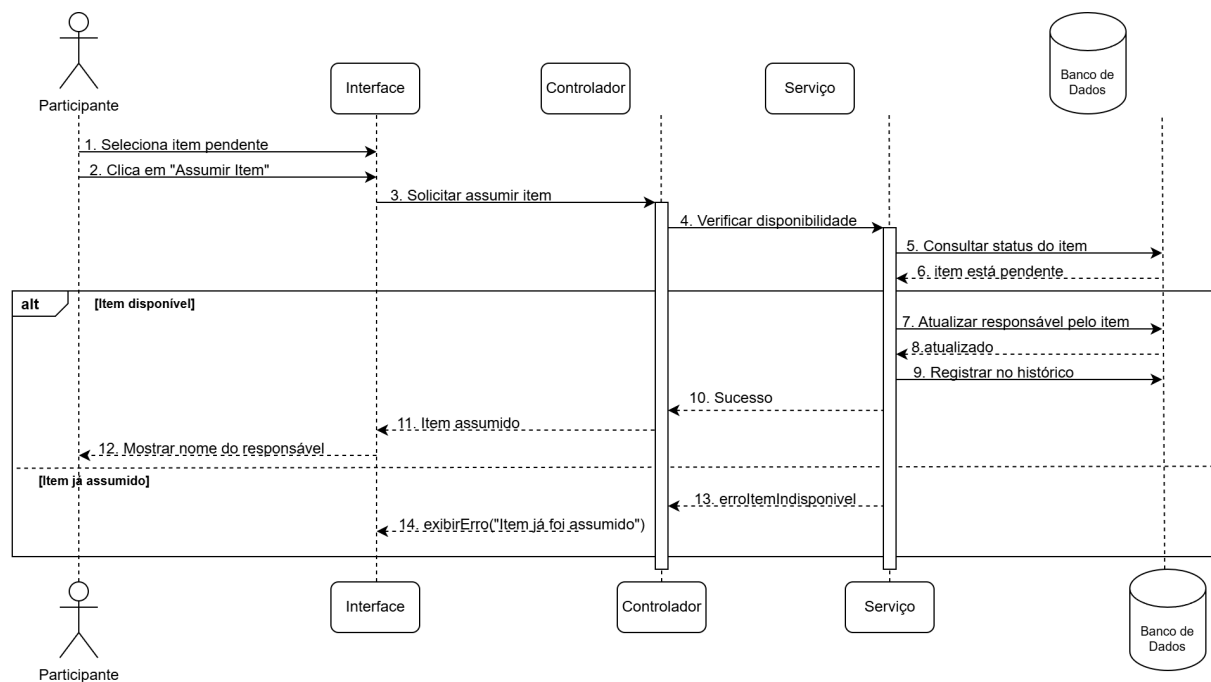
Figura 4 – Sequência Assumir Item.
