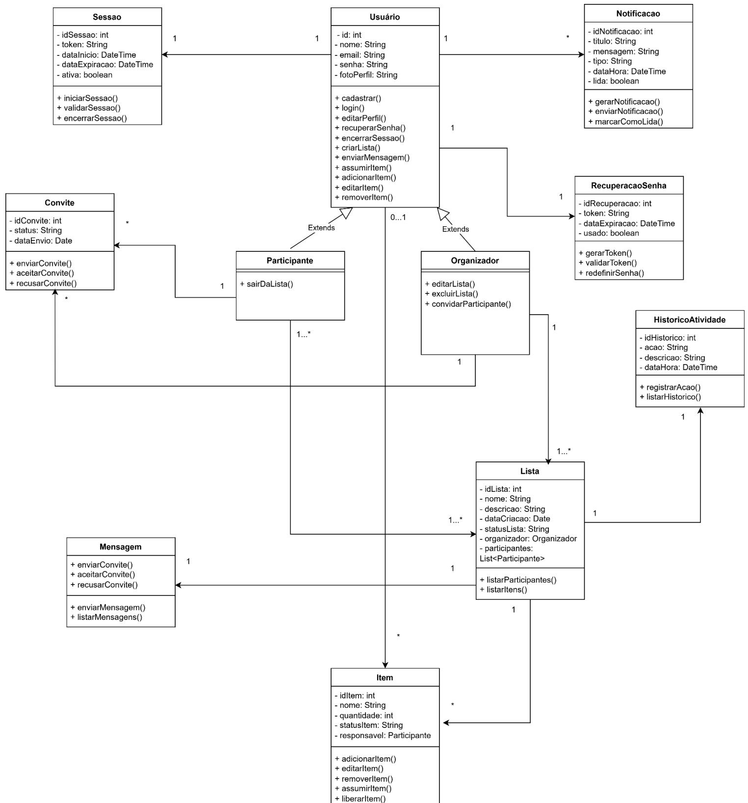
Figura 18 – Diagrama de Classes
