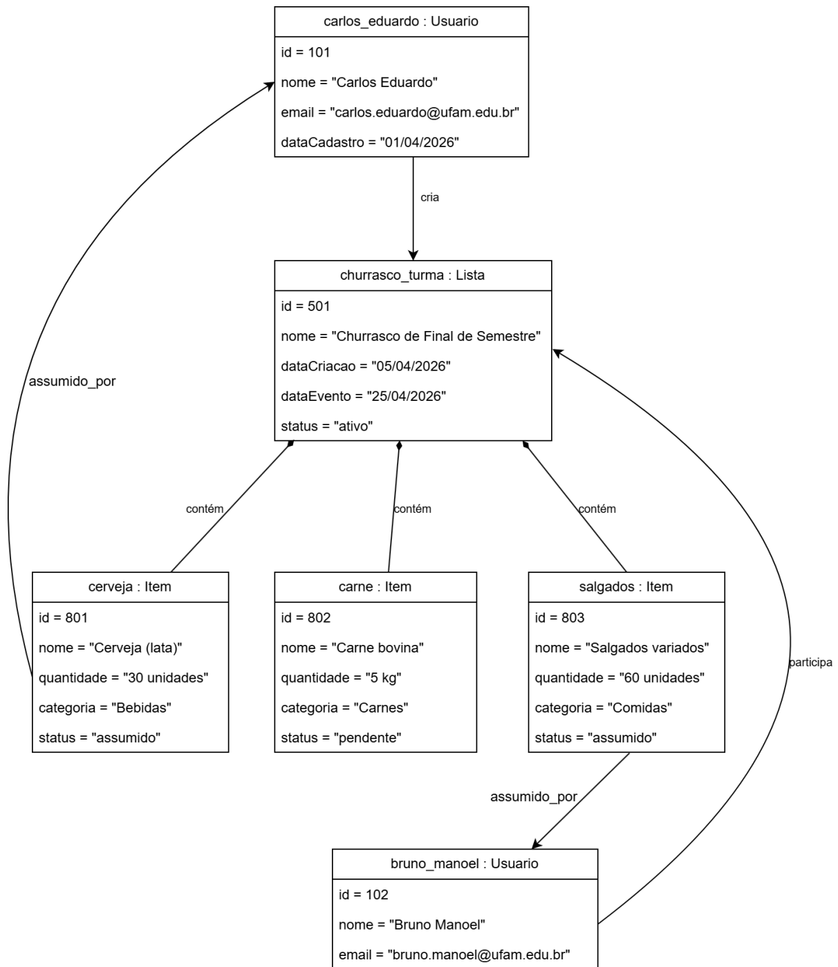
Figura 19 – Diagrama de Objetos
